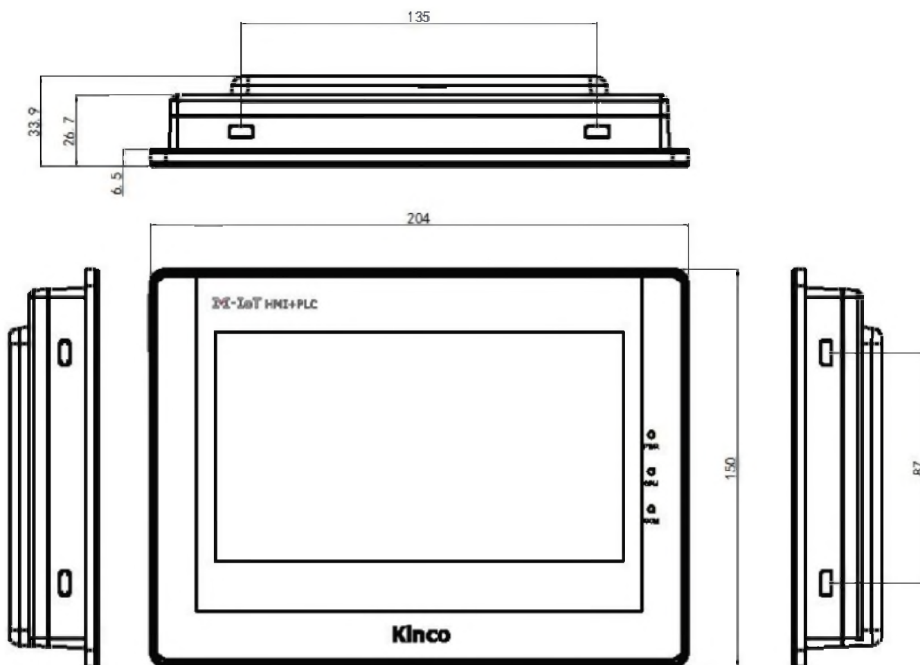
Рис. 2-8 Размеры MK070E
