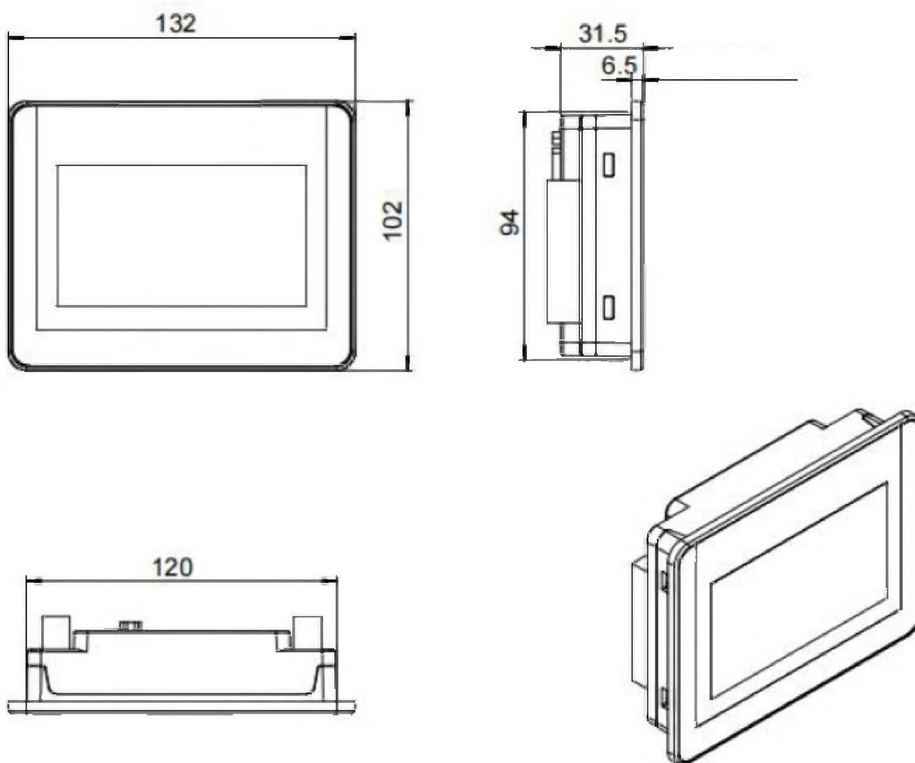
Рис. 2-7 Размеры МК043Е
