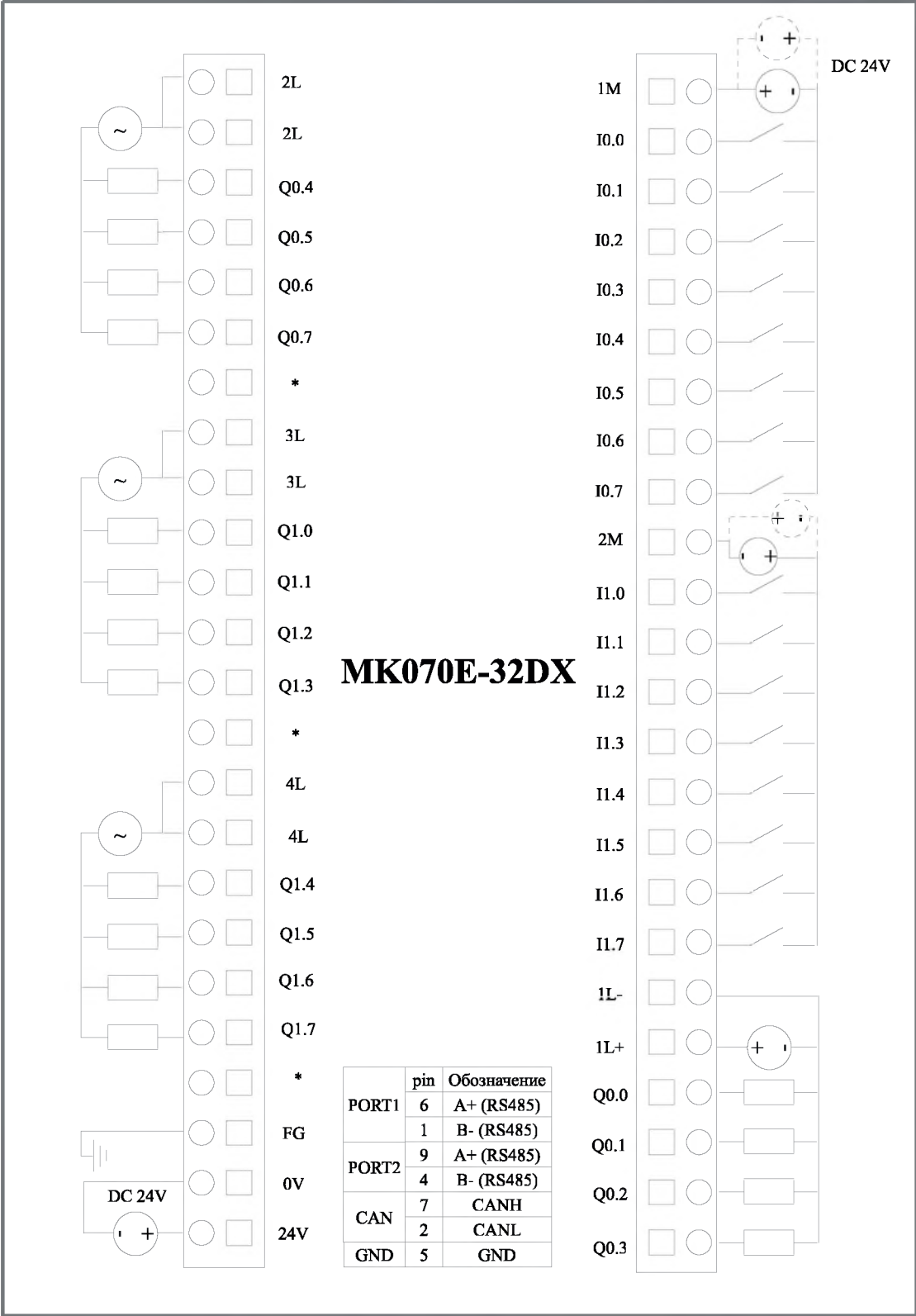
Рис. 2-3 Схема подключения MK070E-32DX
