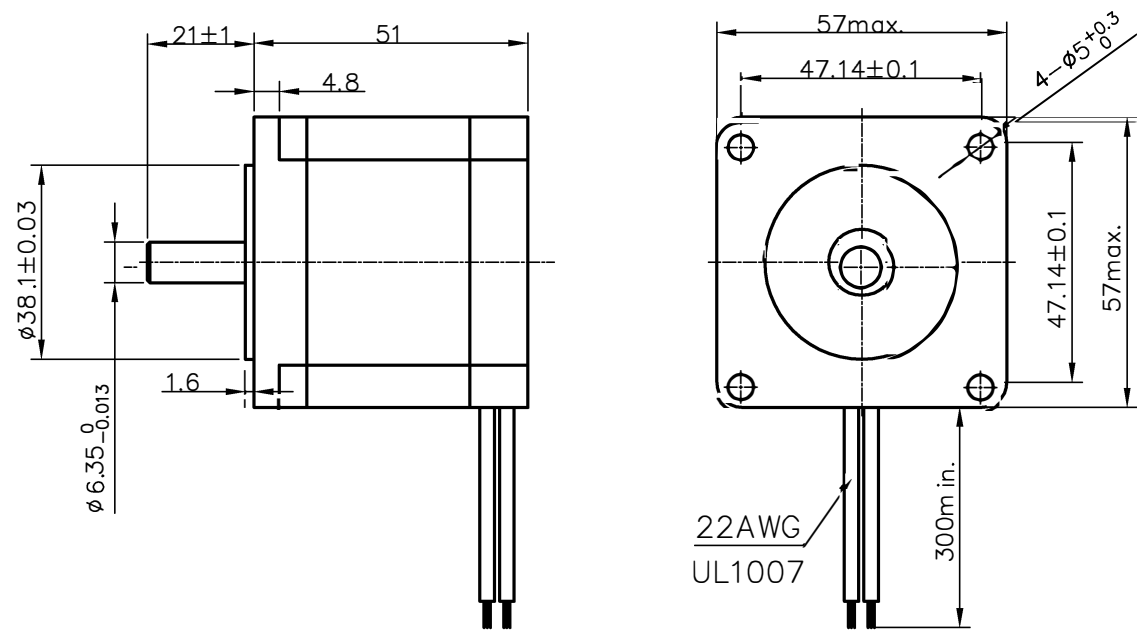
外型图:
