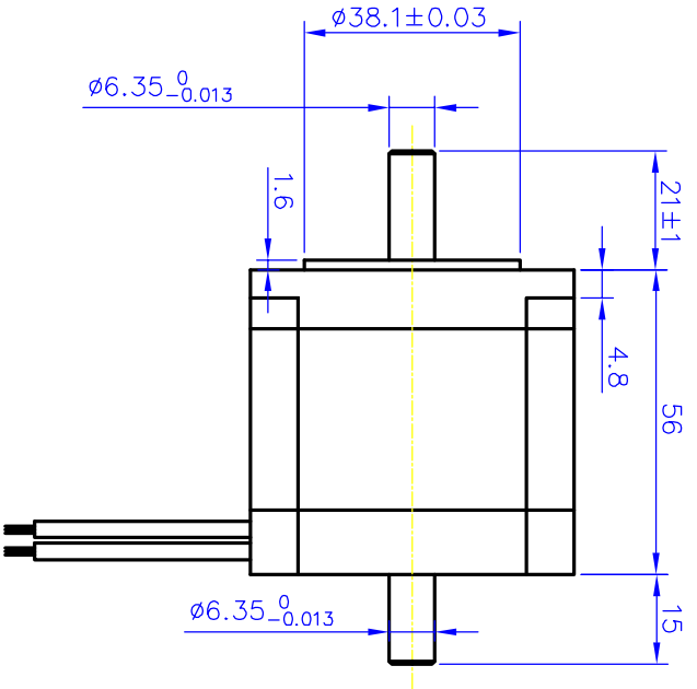
外型图:
